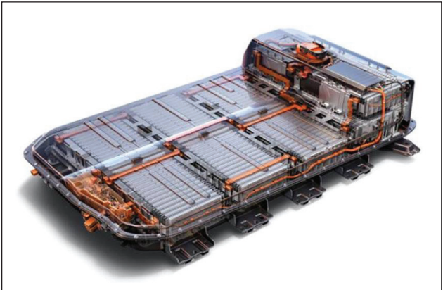
Opbygning af batterier i flere lag, integreret i karosseriet.
