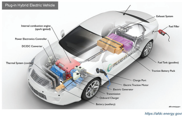
Princip opbygningen af PHEV
