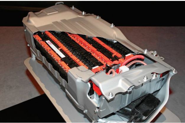
Batteri opbygget i rækker. Tragten til luftkølingen af batteriet fremgår tydeligt nederst til højre.
