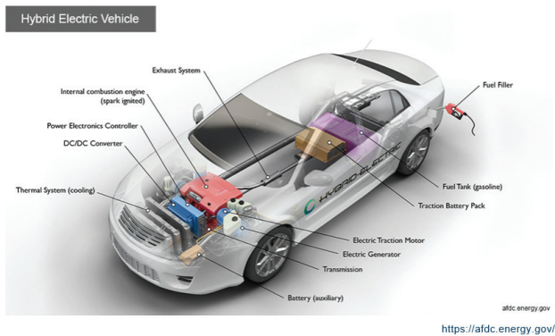
Princip opbygningen af HEV
